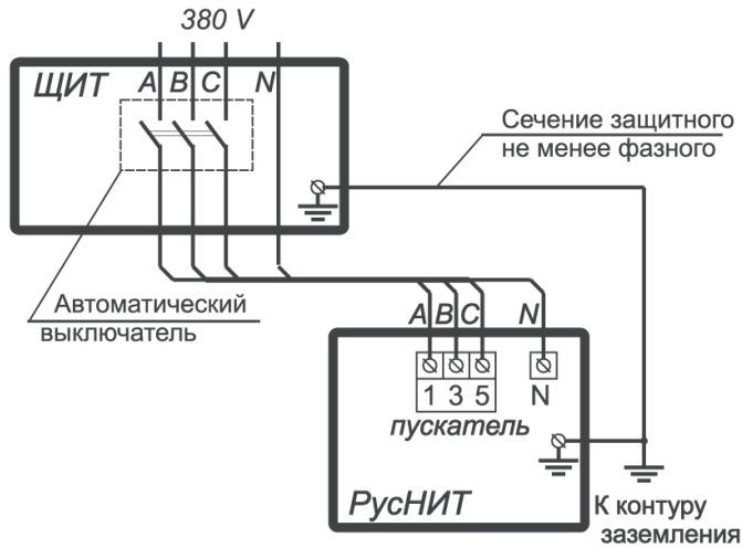
Рис. 6. Схема подключения к трёхфазной сети
